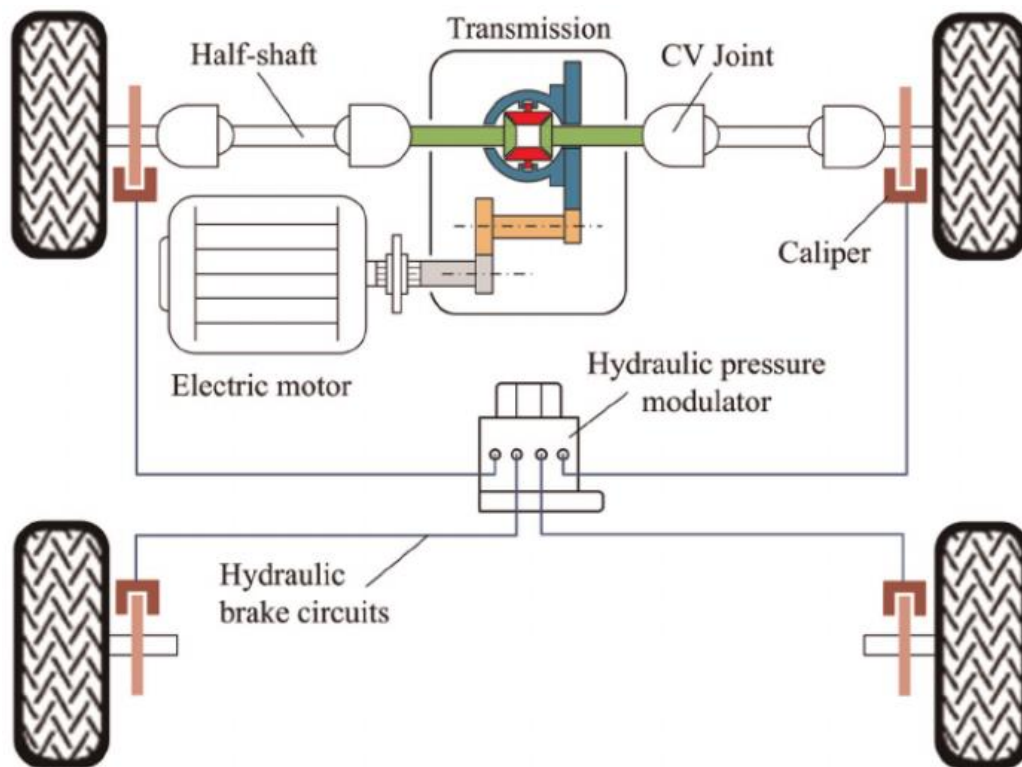
Joonis 2. Elektriauto lihtsustatud blokk skeem [35].
