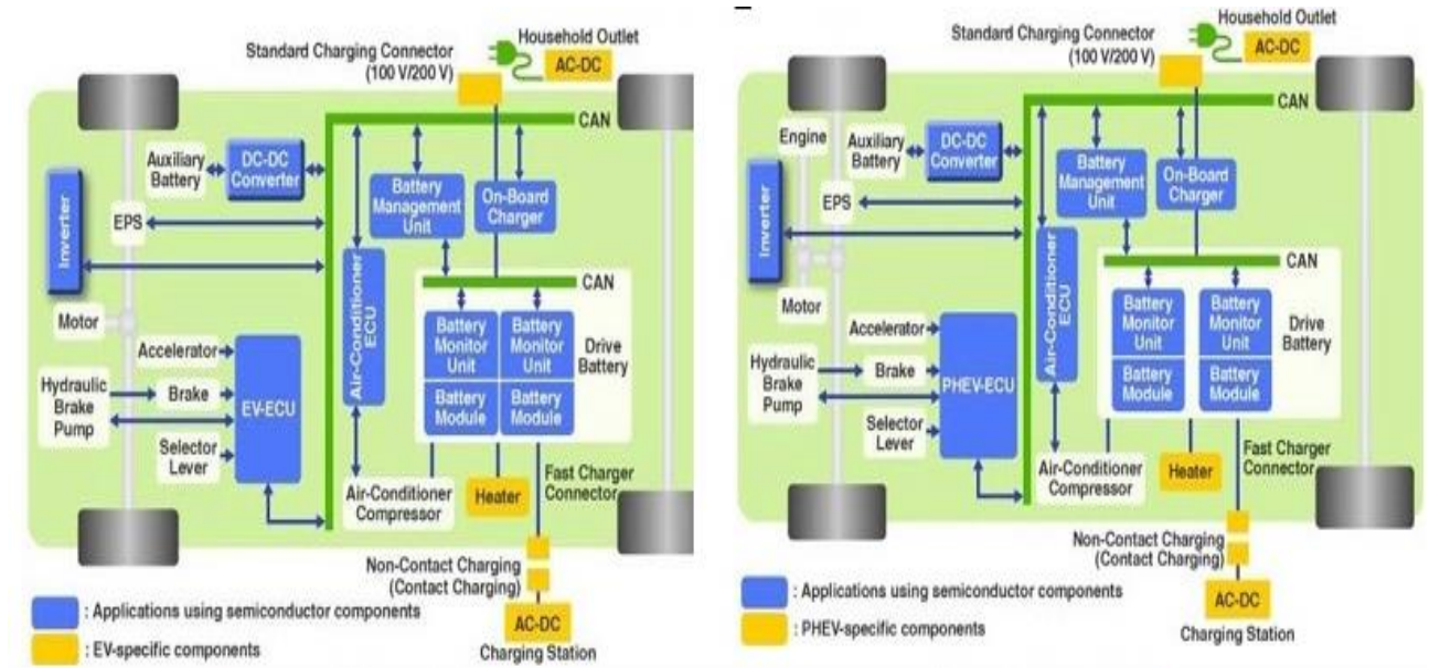
Joonis 1. Vasak pilt illustreerib elektriauto elektrilist blokk skeemi ja parem hübriidauto oma [33].
