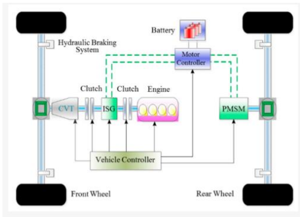
Joonis 3. Lihtsustatud kahemootoriline blokk skeem [34].
