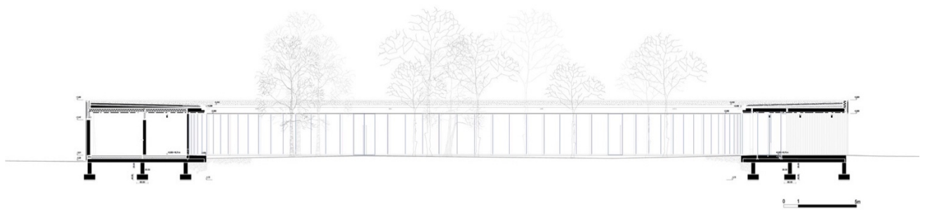
Joonis nr 9. Hostel Vadi lõige. Allikas: Archdaily
