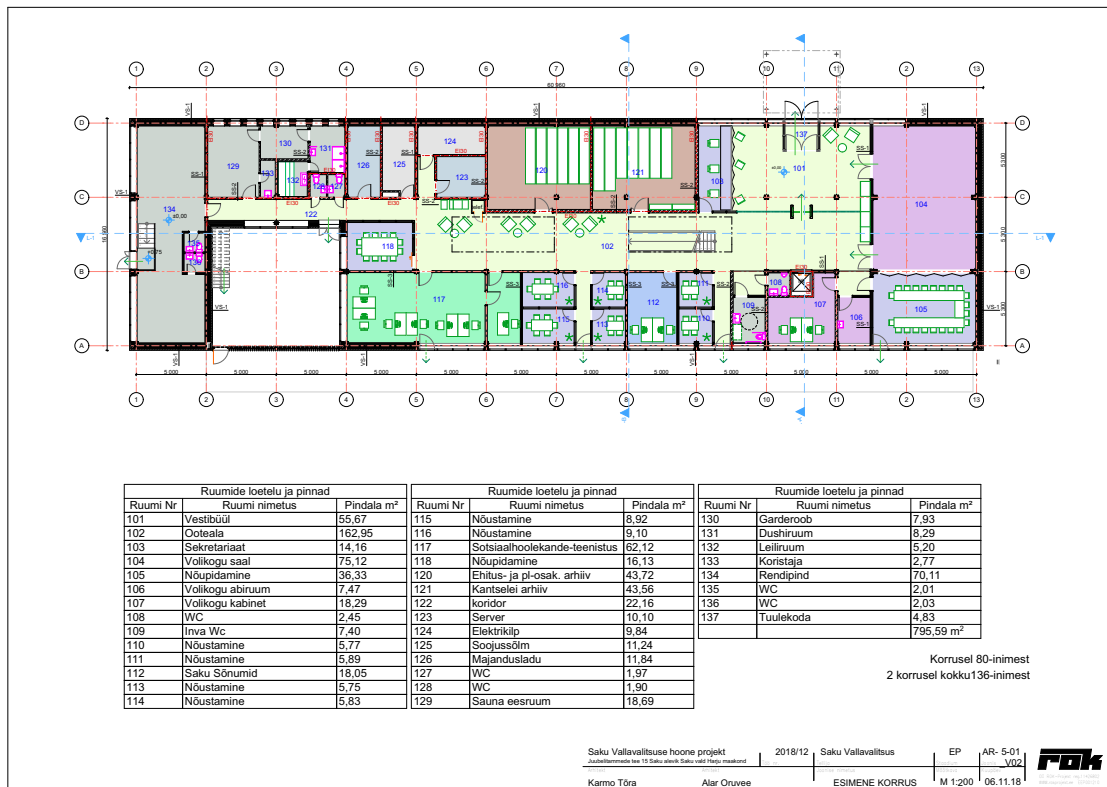
Joonis nr 5. Vallamaja I korrus. Allikas: Ehtisregister
