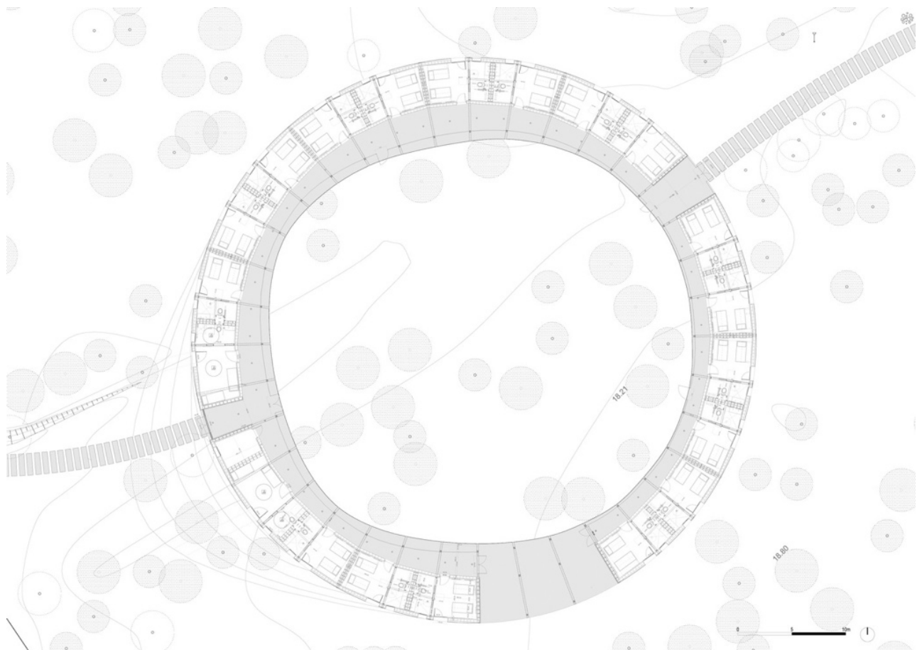
Joonis nr 8. Hostel Vadi plaan. Allikas: Archdaily
